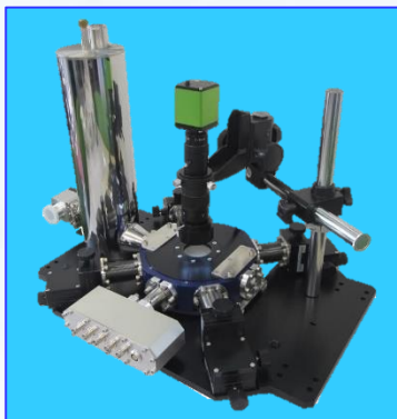
熱電・半導体物性測定プローバ
